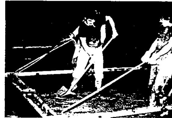
Fig. 29 - Livellamento finale del calcestruzzo mediante staggia vibrante.
